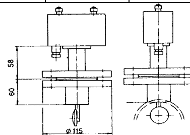
DW - U - AU - FL Przyspawany do rury
