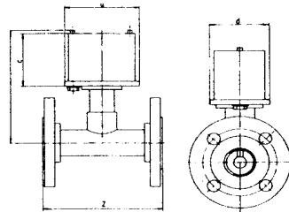
DW - U - FL
